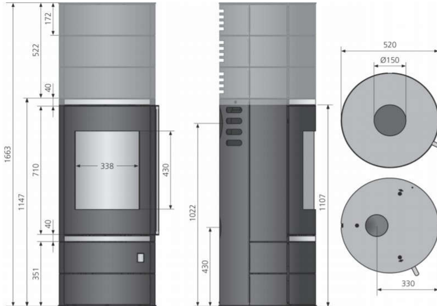
4.7 Maßzeichnung
