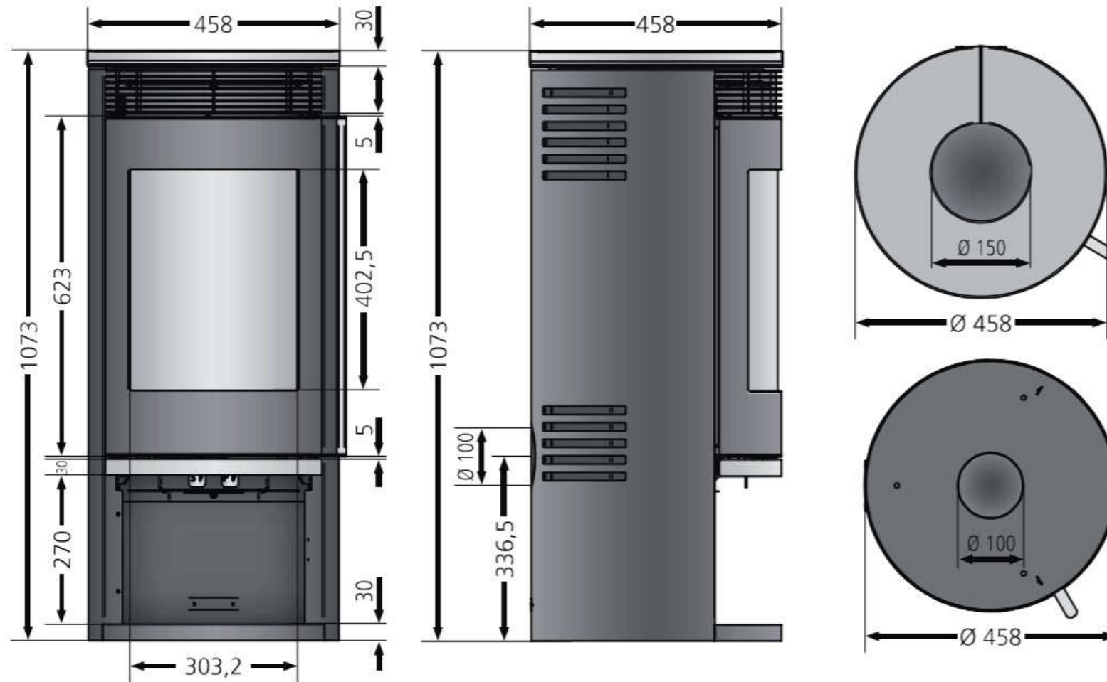
4.7 Maßzeichnung
